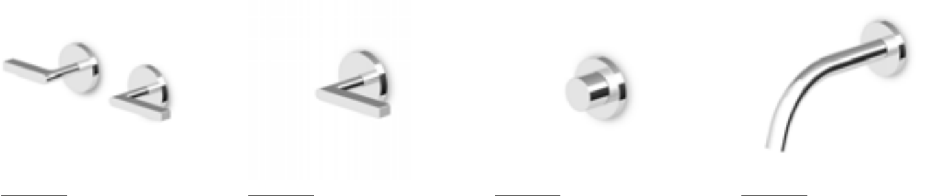
ZSB5738 + R99503 Batteria incasso doccia, rubinetti Hot e Cold Built-in shower mixer, taps Hot and Cold Batería ducha de empotrar, llave hot y llave cold ZSB5729 + R99779 Rubinetto incasso da 1/2” 1/2” wall valve Llave de paso 1/2” Z94540 + R99629 Deviatore da incasso Built-in diverter Desviador de empotrar Z93757 Bocca di erogazione Wall spout Caño
